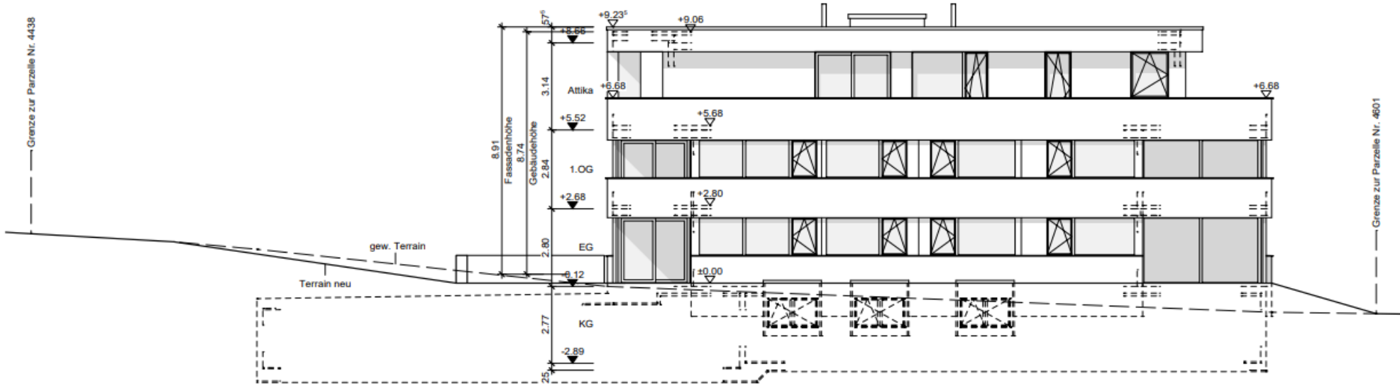
Ansicht Nord-Ost
